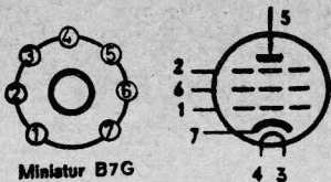
Miniatür B7G
